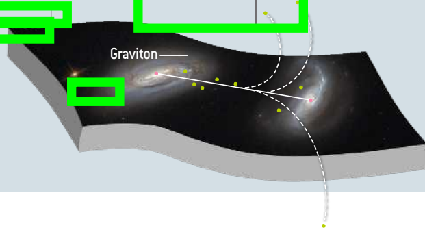
Univers à quatre dimensions Graviton s'échappant dans la cinquième dimension
