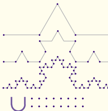
ENSEMBLE BORÉLIEN
