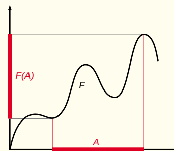
ENSEMBLE BORÉLIEN
