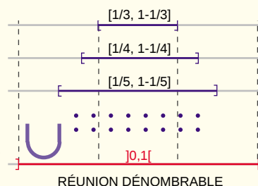
RÉUNION DÉNOMBRABLE
