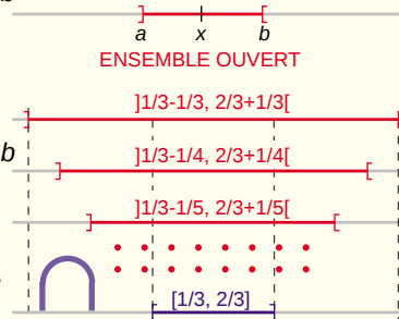
INTERSECTION DÉNOMBRABLE
