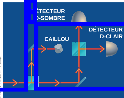
4. DANS L'EXPÉRIENCE de C. Elitzur et L. Vaidman, un photon a le choix entre deux chemins optiques. Les éléments optiques sont disposés de sorte que les photons aillent toujours au détecteur D-clair, et jamais au D-sombre (en haut). Toutefois, la présence d'un caillou sur l'un des trajets envoie parfois un photon sur le détecteur D-sombre (en bas) : une mesure sans interaction a alors eu lieu.
