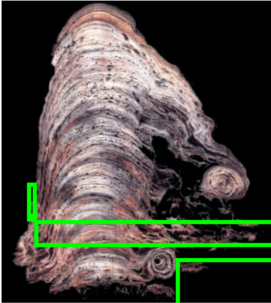
9. STALAGMITE (190 millimètres) incluant deux stalactites fossilisées. La structure interne révèle le développement rythmé, sur 1 500 ans environ, de lamines superposées claires et sombres. Le comptage des lamines permet de dater les chutes des stalactites.
