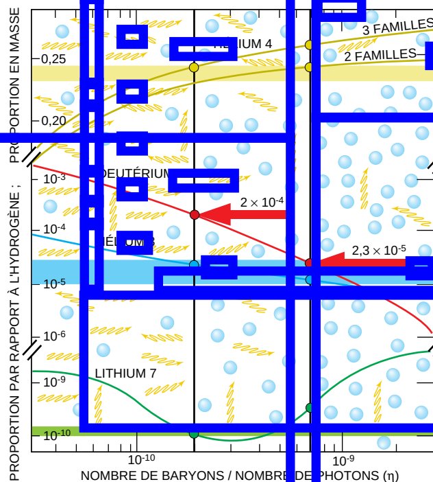
Les deux récentes estimations de la proportion de deutérium primordial (flèches rouges) diffèrent notablement. À partir de chacune de ces mesures, on détermine la quantité de deutérium et d'autres éléments légers produits lors de la nucléosynthèse primordiale. La valeur haute est compatible avec l'ensemble des observations (les bandes jaune, bleue et verte indiquent les mesures des différents éléments légers dans des sites primordiaux, avec les incertitudes de mesures).
