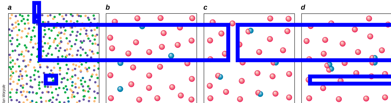
4. LA NUCLÉOSYNTÈSE, ou formation des noyaux atomiques, commença quelques instants après le Big Bang, lors du refroidissement de l'Univers : les quarks (a) s'agglutinèrent en protons et en neutrons (b) ; puis les protons (en rouge) et les neutrons (en bleu) formèrent des paires nommées deutons (les noyaux de deu-
