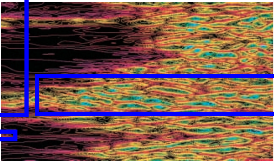
4. CE DÉTAIL DE LA SIMULATION de l'écoulement de l'air sur une aile d'avion (en bas) montre la transition entre un écoulement lisse, laminaire (zones sombres à gauche) et la turbulence (zones ondulantes à droite). On pourrait réduire la traînée en plaçant sur l'aile des microvolets (microphotographie supérieure) qui, se soulevant en fonction des variations de pression, agiraient sur les petits tourbillons qui se forment au voisinage de l'aile.
