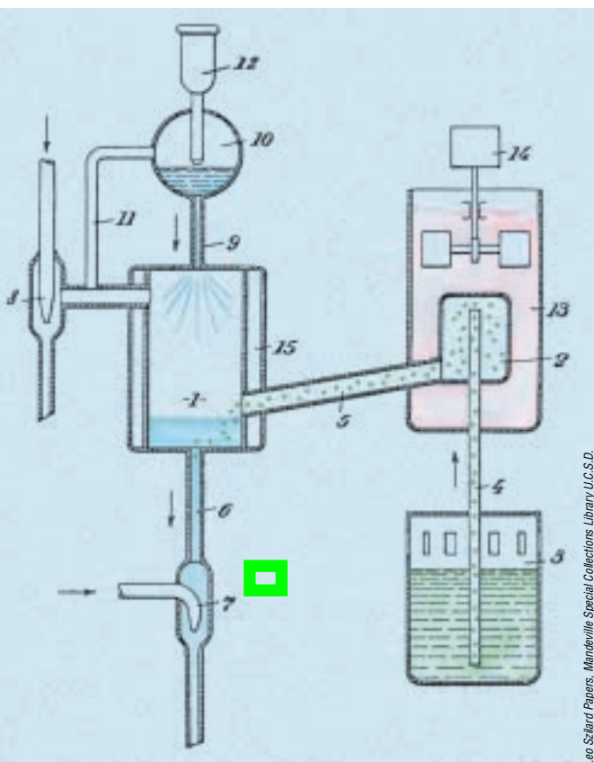
3. LA POMPE À INDUCTION DE L'EAU du robinet devenait actionner ce petit système réfrigérant, construit (après simplification) par la Société Cito-gel, à Hambourg. Le méthanol contenu dans la chambre 1 se vaporisait dans la chambre 2, refroidissant le compartiment 13 qui l'entourait. La turbine 14 délivrait de la crème glacée ou tout autre aliment glacé. Le méthanol, qui se dissolvait dans l'eau de la chambre 1, devait être progressivement remplacé. Le dispositif ne fut pas commercialisé, parce que la pression d'eau fluctuait trop dans les immeubles allemands, vers 1930.
