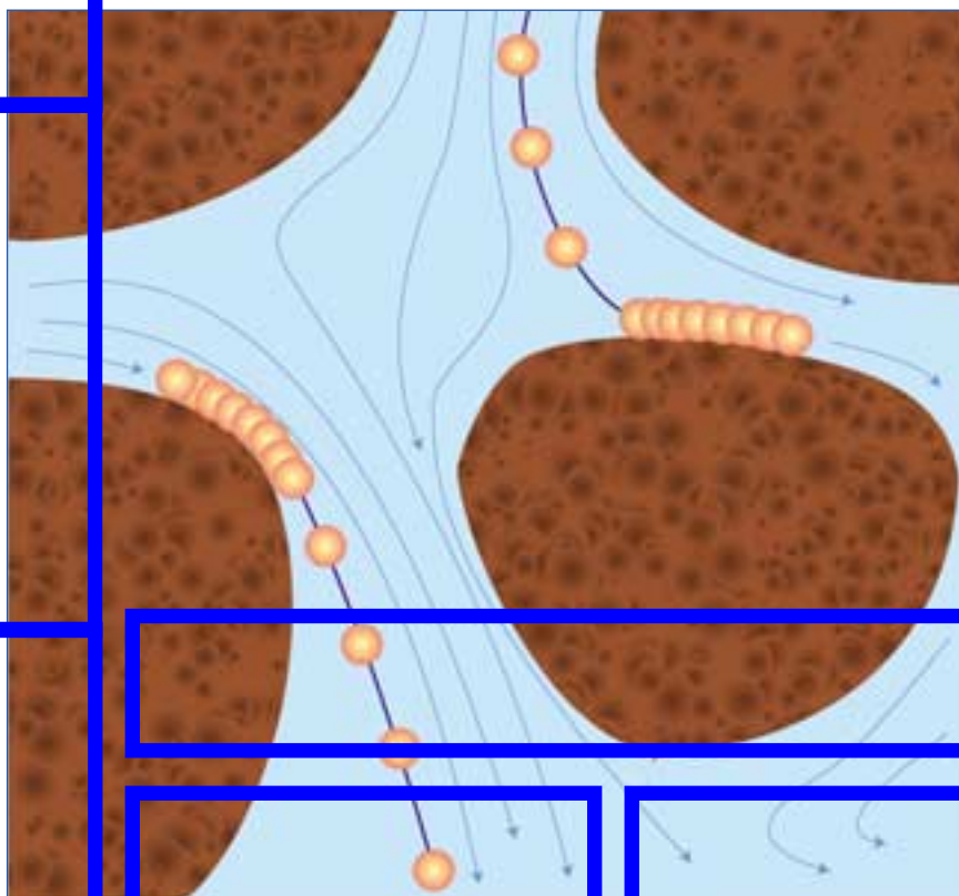
5. DES MOLECULES qui se déplacent rapidement, au centre de l'écoulement dans un pore (en haut), parce qu'elles se trouvent au centre de l'écoulement, peuvent être ralenties, dans le pore suivant, au contact d'un grain. Inversement, des molécules qui se déplaçaient lentement (en bas à gauche), peuvent accélérer. L'effet de dispersion de Taylor n'a donc pas le temps de s'établir.
