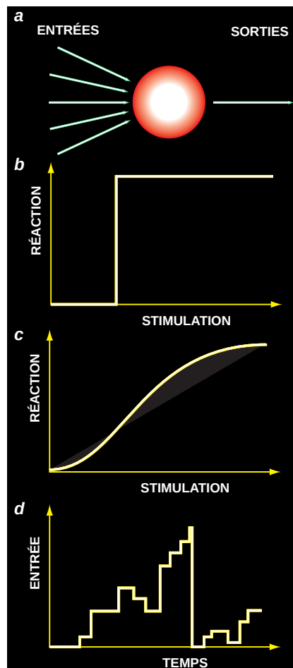
2. DIVERS MODÈLES représentent les neurones de façon plus ou moins réaliste. Les neurones formels de McCulloch et Pitts produisent un signal de sortie égal à 0 ou à 1 selon les signaux d'entrée (b). Les neurones sigmoïdes (c) ont une sortie continue, comprise entre 0 et 1, et d'autant plus proche de 1 que la somme pondérée des entrées est forte. Les neurones «qui intègrent et qui déchargent» (d) calculent la somme des stimulations et des inhibitions au cours du temps et déchargent quand cette somme devient supérieure à un seuil. Le modèle de M. Huxley et M. Hodgkin se fonde sur la physique de la membrane de la cellule nerveuse pour rendre compte des mécanismes d'intégration et d'émission de potentiels d'action.
