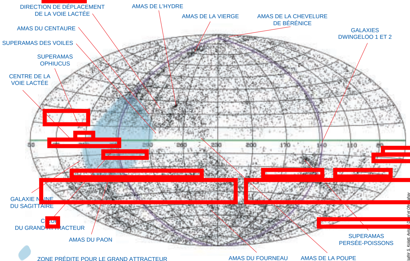
6. TRENTE MILLE GALAXIES , prélevées dans trois catalogues astronomiques classiques, sont représentées par des points sur cette carte. Les galaxies apparaissent partout dans le ciel, sauf dans la zone d'ex-
