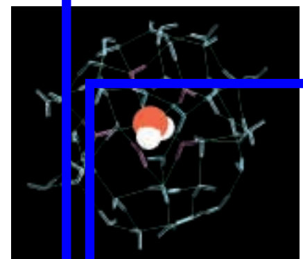
LES LIAISONS HYDROGÈNE confèrent à l'eau ses propriétés particulières. Dans ce modèle, l'eau liquide, la molécule centrale (sphères rouge et blanches) a formé des liaisons hydrogène (lignes vertes) avec cinq autres molécules d'eau (représentées par des V roses). Les atomes d'hydrogène de cette molécule (blancs) se lient à des atomes d'oxygène de deux autres molécules d'eau, et son atome d'oxygène (rouge) est lié à un atome d'hydrogène de trois autres molécules d'eau. Chaque molécule d'eau liquide crée en moyenne 4,5 liaisons hydrogène.
