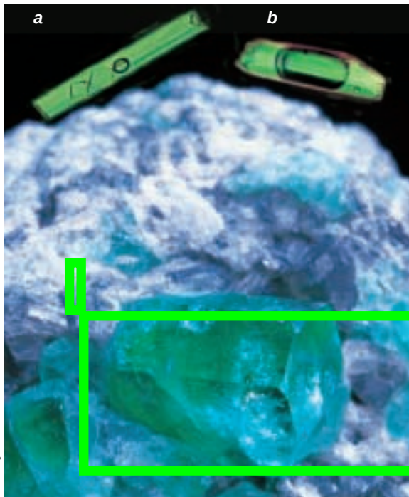
Cristal d'émeraude (en bas) dans sa gangue de carbonates : il mesure environ deux centimètres de longueur et provient d'une mine de Colombie. Les inclusions formées lors de la cristallisation des émeraudes reflètent leur milieu de formation : ainsi, l'inclusion triphasée (a), qui mesure environ 100 micromètres et contient deux cubes de sel (en bas à gauche) et une bulle de gaz (au centre) en suspension dans un liquide, indique une provenance colombienne, tandis que l'autre inclusion (b) révèle une origine bulgare.
