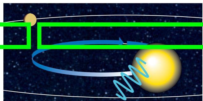
par l'étoile (à droite), en raison de l'effet Doppler (le même phénomène que celui qui décale le son d'une ambulance en mouvement).
