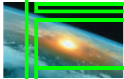
Chute d'une météorite dans l'océan.
