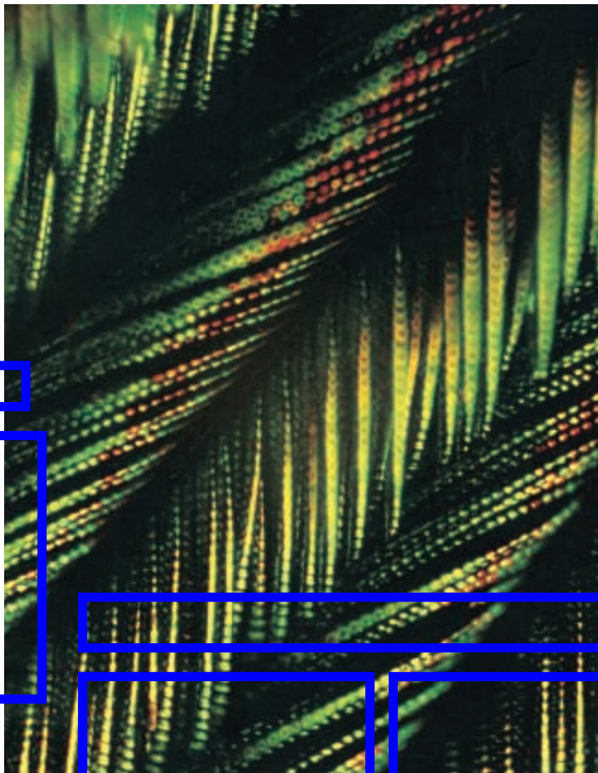
8. PLUME DE PAON observée au microscope optique sur fond noir, avec un éclairage latéral blanc. Les taches colorées correspondent aux cuvettes portées par les barbuies. Les interférences sur les microlamelles des cuvettes engendrent ces couleurs.
