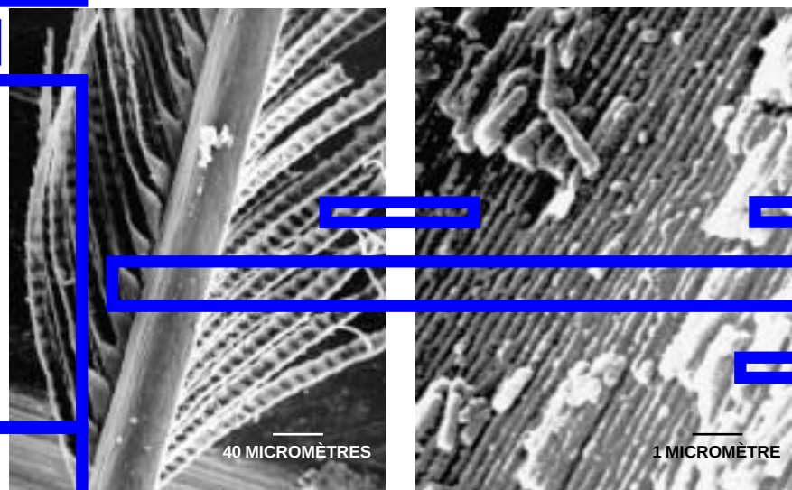
6. BARBULE DE PLUME DE PAON. Chaque barbule renferme une série de cuvettes (flèche jaune). À droite, on voit les microlamelles du fond de ces cuvettes.
