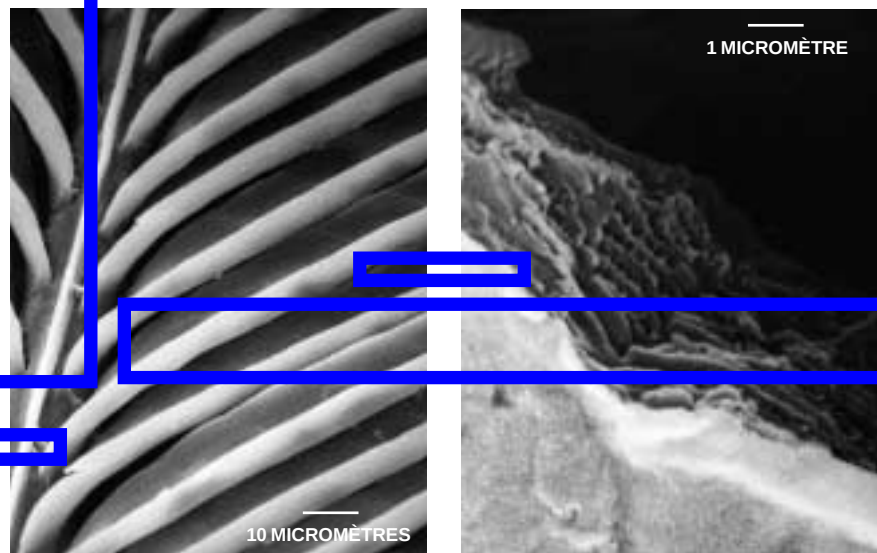
7. SUR LES PLUMES DE COLIBRI (à gauche), les barbules sont pliées suivant leur longueur : on voit ici la face inférieure. Les microlamelles (à droite) décomposent la lumière et engendrent les couleurs.
