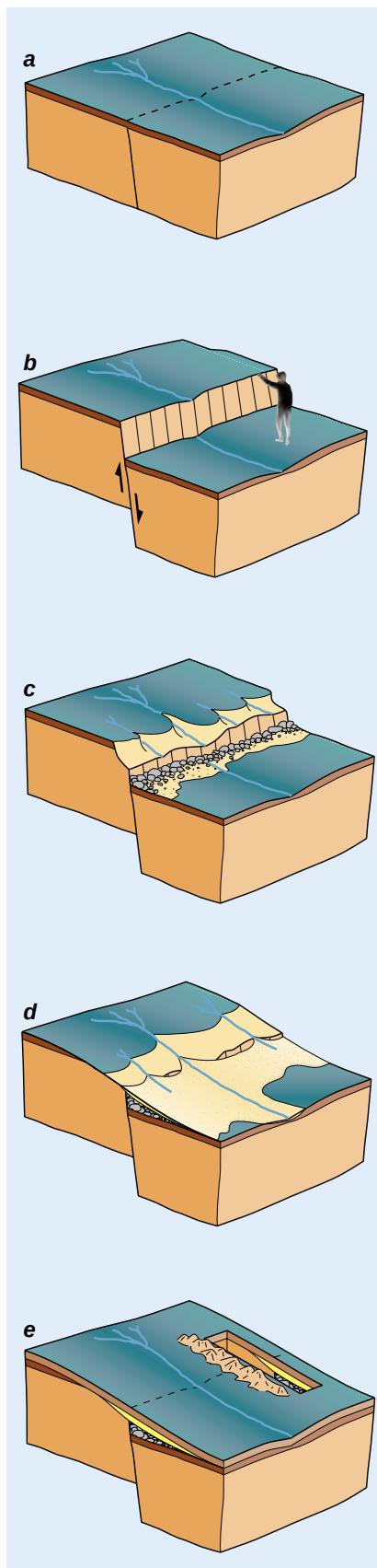
2. ÉVOLUTION D'UN ESCARPEMENT de faille créé lors d'un séisme (b). L'escarpement est progressivement nivelé par l'érosion (c et d). Le paléosismologue creuse une tranchée (e) pour étudier les sédiments issus de l'érosion du compartiment soulevé.
