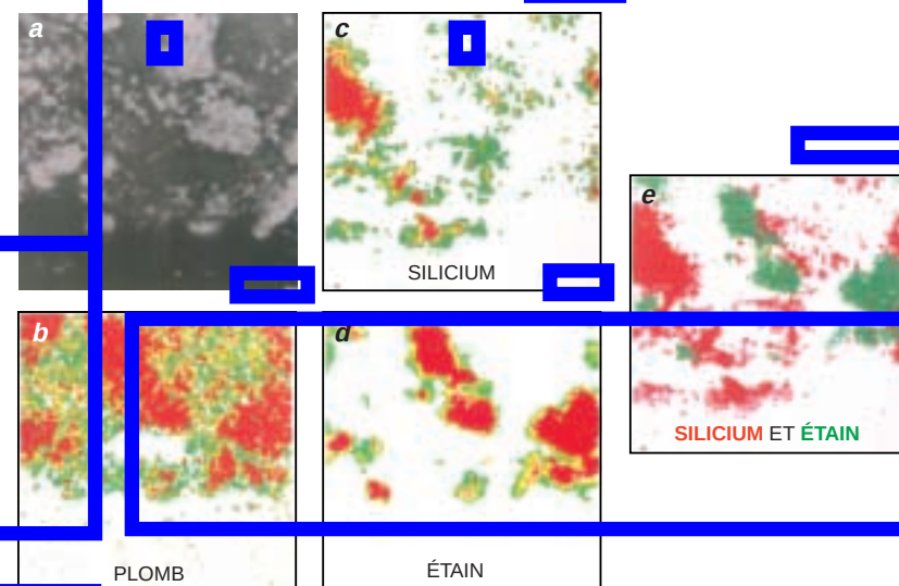
6. ANALYSE DU PORTRAIT DE SIGISMOND MALATESTA, de Piero della Francesca (musée du Louvre), observé au microscope électronique (a). Sur cet échantillon d'une dizaine de micromètres de côté, l'analyse révèle la densité de différents éléments (b, c, d), la densité croissant du vert au rouge. Quelle variété de pigment jaune a été utilisée? Celle constituée essentiellement de plomb et d'étain, ou celle qui contient en plus du silicium? Le fragment contient effectivement du silicium, mais sa répartition n'est pas corrélée avec celle de l'étain (e) : ils n'appartiennent donc pas au même pigment. C'est la première variété qui a été utilisée et le silicium provient ici d'un pigment ocre.
