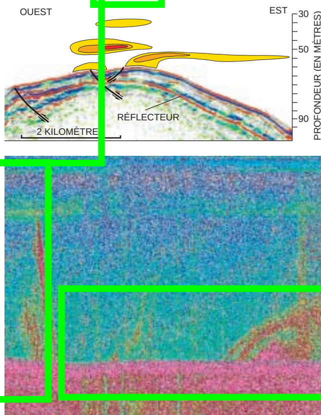
6. ON A DÉTÉCTÉ des panaches de méthane dans l'eau de mer au-dessus de failles (lignes noires avec flèches dans le schéma supérieur). Dans le profil sismique du plancher océanique, la limite inférieure de la couche d'hydrates de gaz est clairement visible sous forme d'un réflecteur. Les zones jaunes, orange et rouges, dans l'image supérieure, indiquent des concentrations respectivement égales à 5, 10 et 50 nanolitres par litre. Un sonar utilisé pour la détection des bancs de poissons a identifié des panaches de méthane qui s'élevaient du plancher océanique dans la mer d'Okhotsk (en bas).
