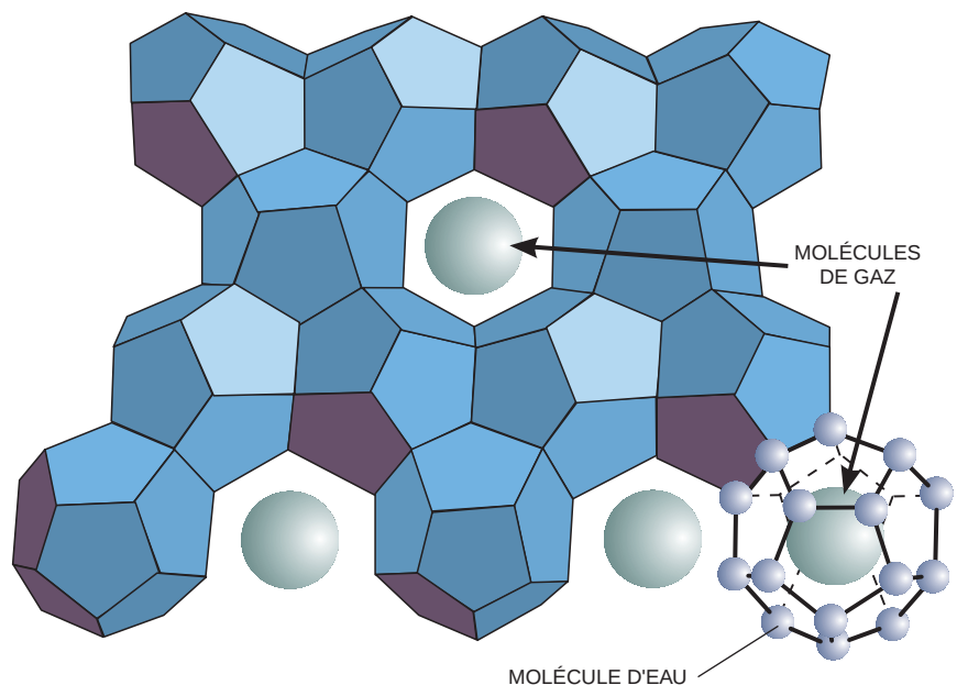
5. DES MOLÉCULES D'EAU forment des cages dodécédriques (en bas à droite) dans les hydrates de gaz. Ces cages piègent des molécules de gaz variés, tels le méthane ou le sulfure d'hydrogène.
