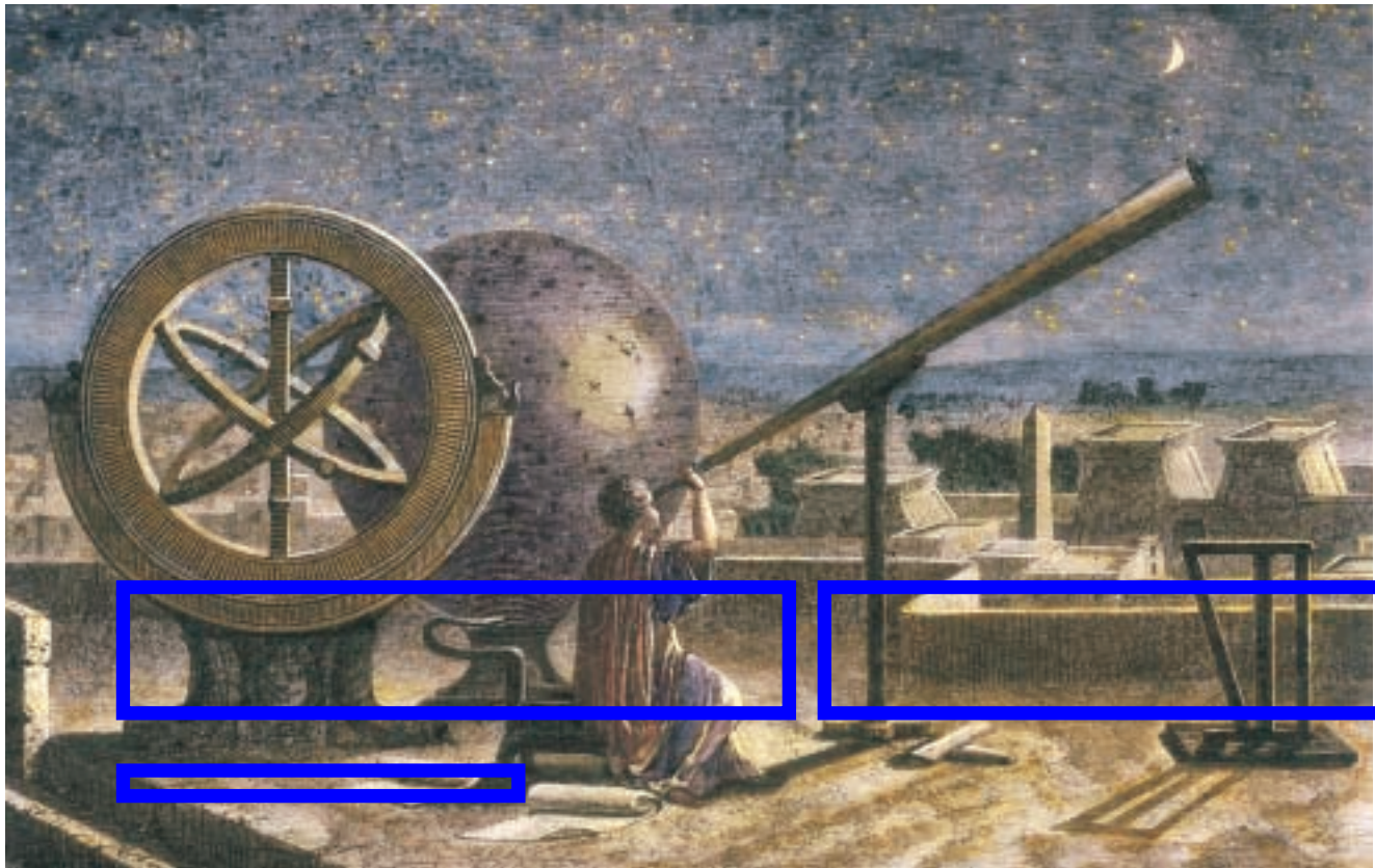
Hipparque dans son observatoire d'Alexandrie : sur cette représentation, la lunette astronomique découverte à la fin du xvi^e siècle est anachronique ; en revanche, les Grecs utilisaient bien les sphères armillaires (à gauche). En l'an -260, Aristarque de Samos estima, par un raisonnement géométrique simple, que le Soleil devait être beaucoup
