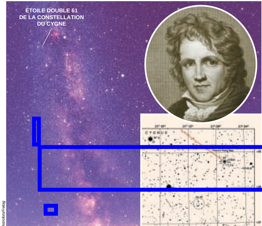
Friedrich Wilhelm Bessel fut le premier, en 1838, à déterminer la parallaxe d'une étoile et, par conséquent, sa distance à la Terre ; il s'agissait de l'étoile double 61 de la constellation du Cygne. Sa distance a été déterminée à nouveau par le satellite HIPPARCOS : elle est égale à 11,4 années-lumière, et cette étoile double se déplace de 1,5 degré au firmament, en l'espace d'un millénaire (flèches sur la carte stellaire ci-dessus), valeur qui correspond à trois fois le diamètre de la Lune.
