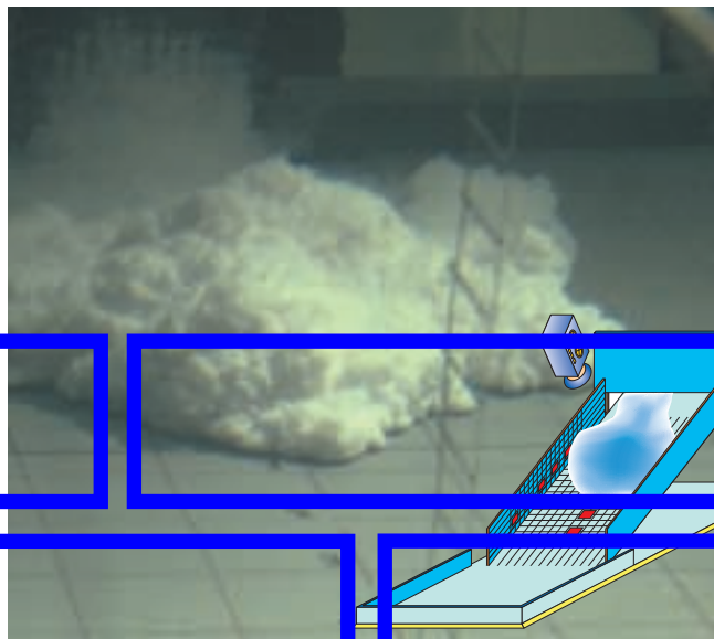
9. PAR DES EXPÉRIENCES EN LABORATOIRE, on mesure les paramètres des modèles numériques. Une masse de neige artificielle est libérée par une trappe sur un plan incliné muni de capteurs (en rouge sur le schéma) et filmé par une caméra. Dans un autre type d'expériences, les écoulements aérosols sont simulés par des suspensions de particules dans un bassin rempli d'eau (photographie).
