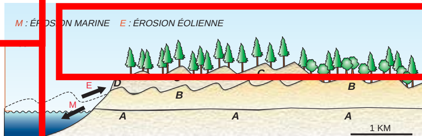
1. Coupe Ouest-Est de la côte du littoral aquitain. Le sable des Landes (A) a été déposé par le vent pendant la dernière époque glaciaire. Les dunes paraboliques (B) se sont formées il y a 5 000 à 2 000 ans, à une époque où le sable était abondant. Les dunes modernes (C) sont apparues à l'époque gallo-romaine, et ont été fixées par une forêt de pins au XIXe siècle. Ainsi la côte est modelée par l'érosion marine (M) et par l'érosion éolienne (E), qui attaquent le bourrelet dunaire (D).
