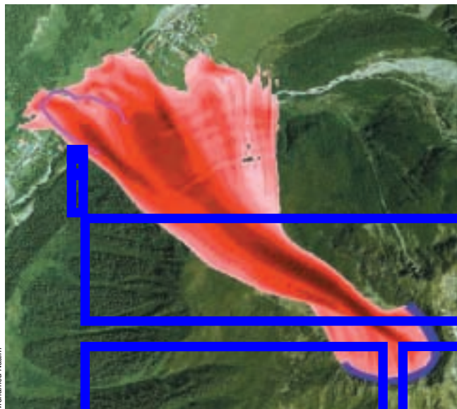
8. LA SIMULATION NUMÉRIQUE de l'avalanche de Montroc, près de Chamonix, en Haute-Savoie, montre l'onde de pression (plus le rouge est foncé, plus la pression est forte) de la neige détachée de la zone de départ (en bleu, en bas à droite). L'écoulement dense, dont la zone d'arrêt, dans le village même, est marquée en violet, a suivi deux couloirs différents.
