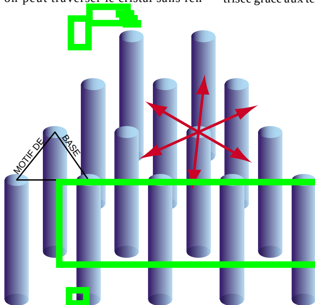
5. UN CRISTAL PHOTONIQUE BIDIMENSIONNEL est constitué d'un assemblage de tiges diélectriques cylindriques séparées par de l'air. Le motif périodique est un triangle équilatéral, et la structure possède une symétrie hexagonale : la lumière se propage de manière identique dans les six directions (flèches rouges). Grâce à cette symétrie, si la transmission de la lumière est interdite suivant une direction, elle le sera pour les cinq autres.
