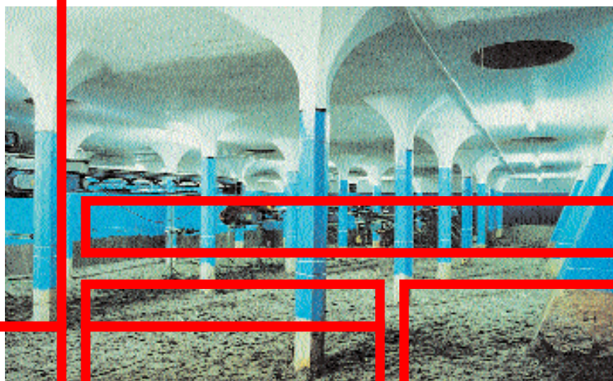
8. LES COLONNES ÉVASÉES de l'immeuble Filter (construit par Maillart en 1912, à Rorschach, en Suisse), se fondent dans le plafond, c'est-à-dire dans les dalles de l'étage supérieur, qu'elles soutiennent à elles seules, sans poutres horizontales.
