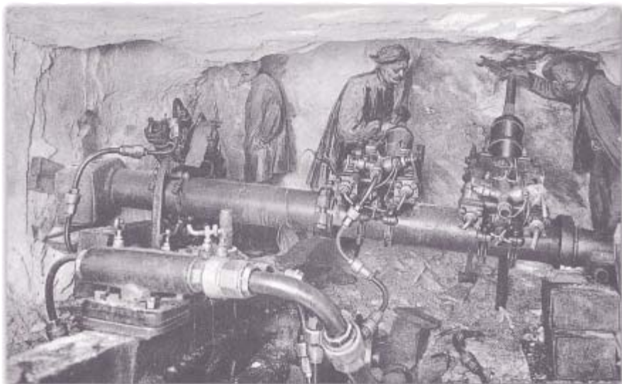
3. Cette foreuse hydraulique a facilité les travaux de percement du tunnel du Simplon, au début du XX e siècle. Elle pouvait réaliser trois trous de mine en même temps.
