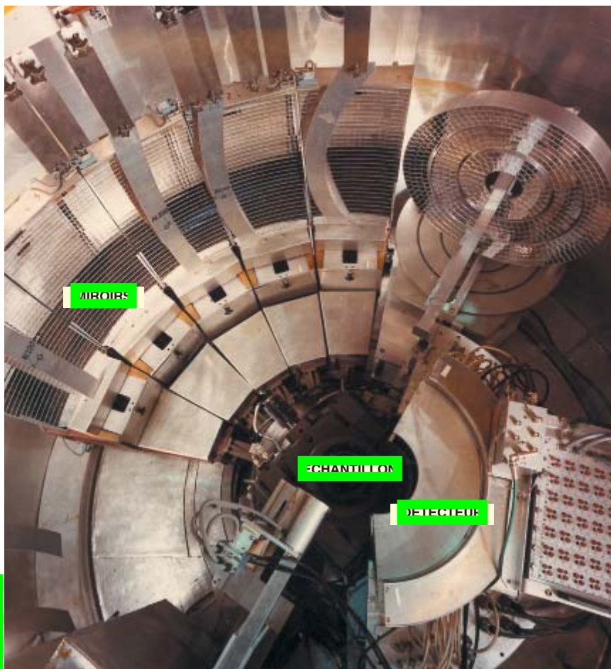
5. LA MESURE DE L'EFFET TUNNEL est fondée sur la diffusion des neutrons (ici, un spectromètre de rétrodiffusion à l'Institut Laue Langevin). L'échantillon, placé au centre de l'enceinte d'environ trois mètres de diamètre, est entouré de miroirs où se réfléchissent les neutrons avant d'être captés par le détecteur.
