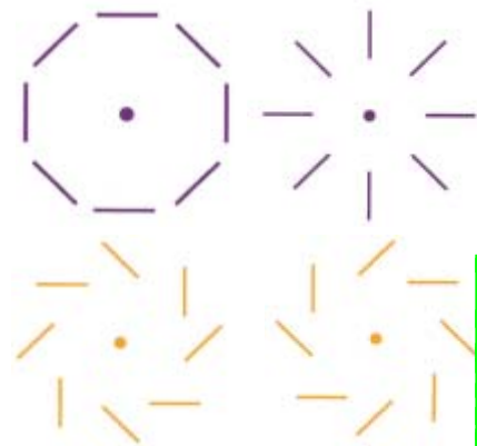
5. LA POLARISATION du rayonnement cosmologique diffus devrait nous renseigner sur les premiers instants de l'Univers. Des fluctuations de densité du plasma primordial auraient créé des motifs de polarisation en anneau ou en étoile ( en haut ) ; les ondes gravitationnelles, au contraire, auraient produit des tourbillons gauches ou droits ( en bas ).
