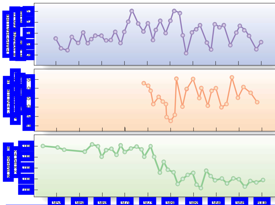
3. EVOLUTION DES PARAMETRES DEMOGRAPHIQUES du manchot empereur de la terre Adélie. Dans les années 1970, au cours d'une période chaude anormalement longue (en haut), la population des manchots a notablement diminué (en bas). Durant cette période, l'étendue de la glace de mer était réduite (au milieu). Aujourd'hui, la population de ce manchot s'est stabilisée.
