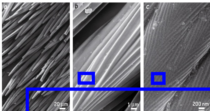
4. À L'ÉCHELLE MACROSCOPIQUE, les poils du coléoptère Celerostoma pinnosa sajjara sont désordonnés (a), puis la structure devient fractale à plus petite échelle. Chaque poil est structuré par un réseau de chevrons (b), et chaque chevron de même (c). Ce désordre structurel à plusieurs échelles optimise à la fois son hydrophobie et sa rigidité.
