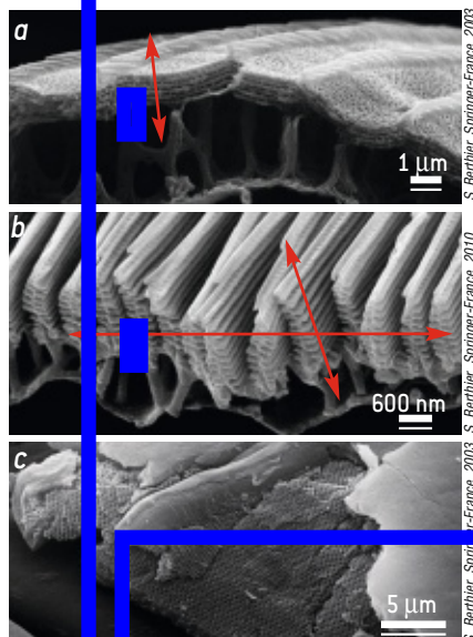
2. TROIS EXEMPLES de structures photoniques chez les insectes : la structure unidimensionnelle de l'écaïlle du lépidoptère Urtica leilus (a), la structure bidimensionnelle de l'écaïlle du lépidoptère Morpho rhetenor (b) et la structure tridimensionnelle de l'écaïlle du coléoptère Cyphus hancoki (c).
