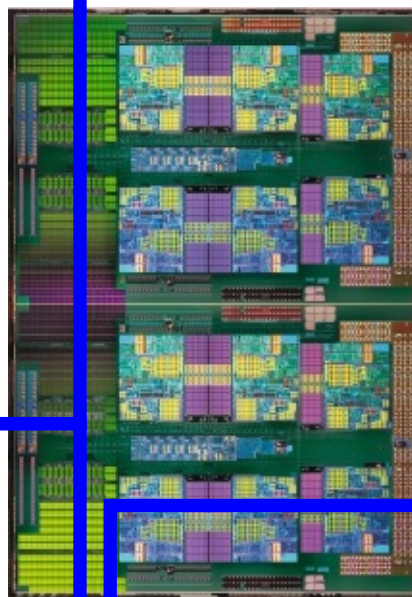
LE PROCESSEUR OPTERON 6100 D'AMD, ici sur une image légèrement agrandie, réunit deux circuits intégrés qui contiennent au total plus de 1,8 milliard de transistors. Les couleurs correspondent aux différents blocs fonctionnels.
