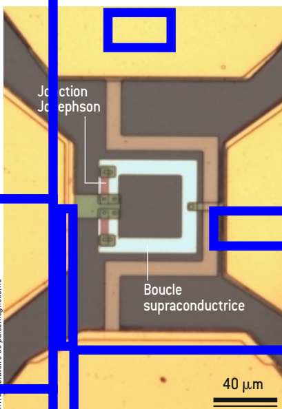
5. LA MAGNÉTOENCÉPHALOGRAPHIE consiste à enregistrer les infimes champs magnétiques produits par l'activité du cerveau. Pour cela, le patient porte un casque (en haut) tapissé de centaines de petits capteurs à base de SQUID. Un SQUID est un circuit supraconducteur très sensible au champ magnétique qui le traverse (ci-dessus).
