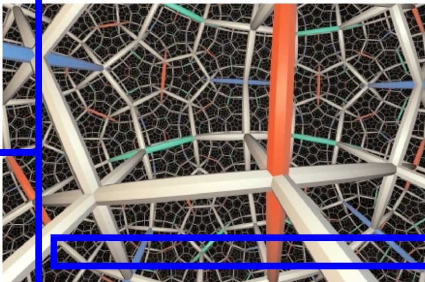
7. L'INTÉRIEUR D'UNE BOULE HYPERBOLIQUE pavée d'une façon régulière par des dodécaèdres. Les couleurs n'ont pas de signification particulière dans cette représentation artistique du pavage.
