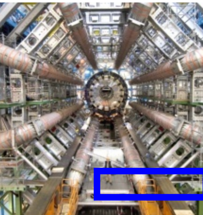
Le détecteur ATLAS lors de sa construction.
