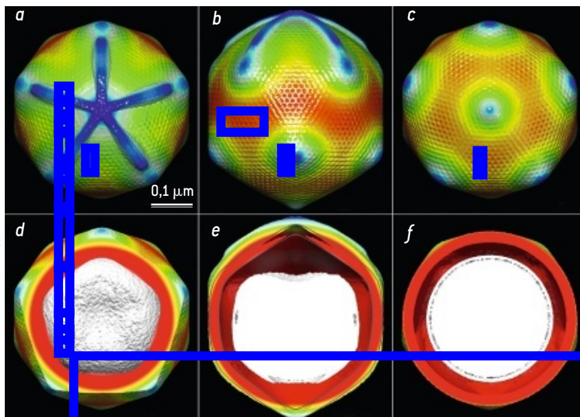
4. UNE RECONSTRUCTION DE LA STRUCTURE DU MIMIVIRUS sans les fibres, d'après des images de cryomicroscopie électronique, sous trois angles différents (d, e, f sont des vues en coupe). Les couleurs traduisent la distance radiale à partir du centre du virus : gris entre 0 et 180 nanomètres, rouge entre 180 et 210 nanomètres, couleurs de l'arc-en-ciel entre 210 et 250 nanomètres.
