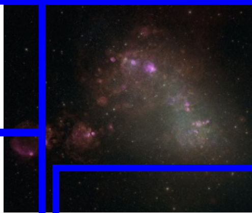
Le milieu interstellaire du Nuage de Magellan (ci-dessus) contient du lithium dans des proportions compatibles avec la théorie de la nucléosynthèse primordiale.
