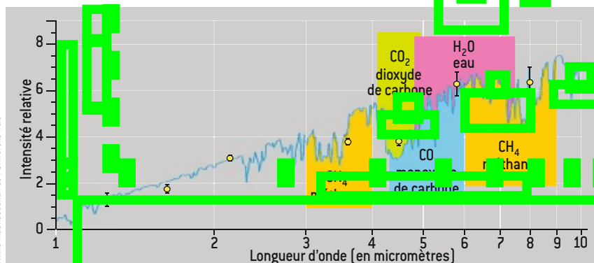
4. LE SPECTRE D'UNE EXOPLANÈTE , le cas d'un jupiter chaud, WASP-12b, permet d'étudier la composition chimique de son atmosphère. Certaines raies (points jaunes) sont compatibles avec un modèle de spectre d'émission (courbe bleue).
