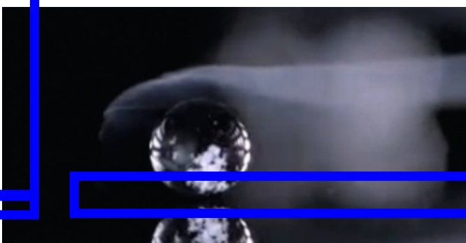
Une goutte d'azote liquide en lévitation sur une surface chaude. Elle est sustentée par la vapeur émise au niveau de sa face inférieure.
