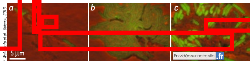
Après traitement à l'isoniazide (a) et avant un nouveau traitement (b), les bactéries M. smegmatis résistantes (en vert) se multiplient (b).
