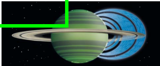
Les particules chargées des anneaux tomberaient sur Saturne le long des lignes de champ magnétique (en bleu), ce qui ferait disparaître certains éléments de la haute atmosphère (bandes sombres).
