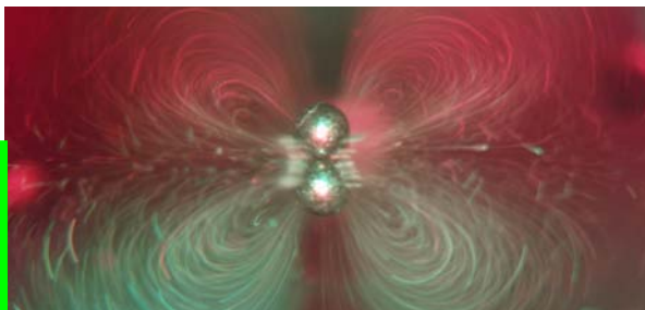
Le coulement entre les billes crée un mouvement de rotation
