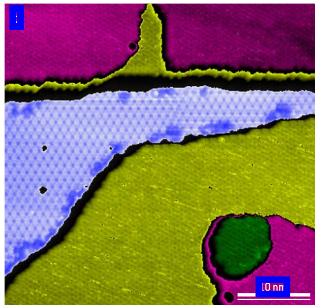
2. LES IMAGES DU SILICÈNE au microscope à effet tunnel révèlent des caractéristiques variées de ce matériau. On observe les domaines dont l'orientation des mailles diffère [a, les zones bleues entourées de rouge]. La méthode permet aussi de visualiser les empilements de plusieurs couches de silicène [b, en bleu, vert, rose et vert foncé].
