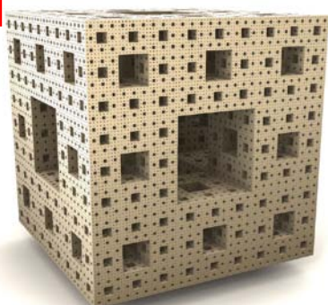
éponge de Menger IM
