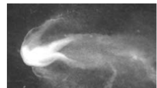
Au tout début de son développement, l'embryon de poulet se replie sur lui-même et délimite le tube neural (à droite, de haut en bas, images séparées de 100 minutes). Ci-dessus, l'embryon dix jours plus tard.
