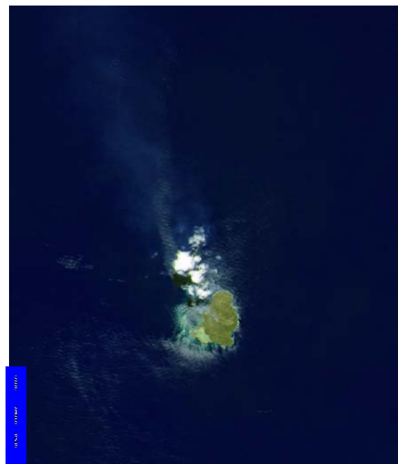
NAISSANCE D'UNE ÎLE : exemple de volcanisme sous-marin, l'île de Nishino-shima shinto a émergé de la surface du Pacifique en novembre 2013. Émettant sans cesse des laves, elle a grossi jusqu'à toucher l'île voisine de Nishino.
