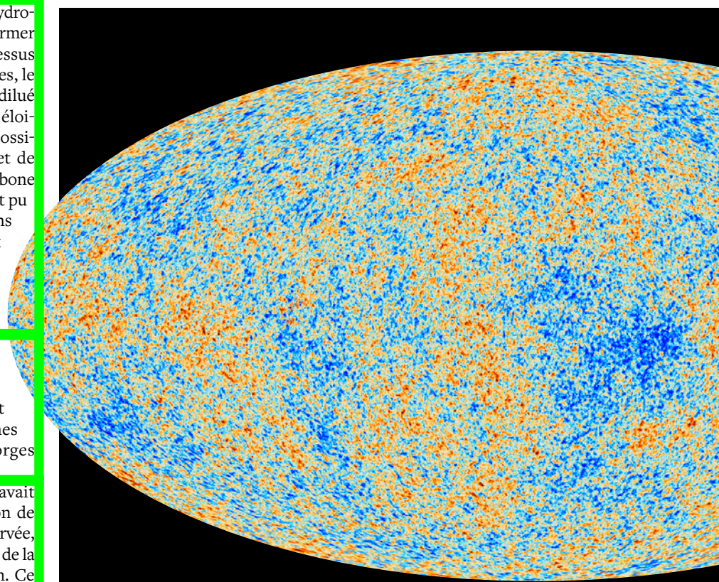
Les fluctuations de température du fond diffus cosmologique enregistrées par Planck évoquent des conditions qui régnaient dans l'Univers lorsqu'il était âgé de 380 000 ans.
