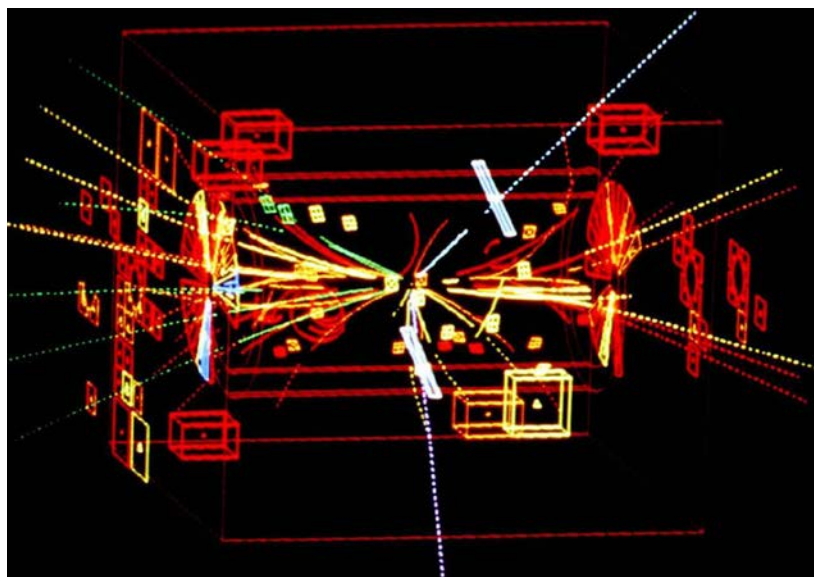
Reconstruction numérique de la désintégration d'un boson Z en un électron et un positron enregistrée le 30 avril 1983. Il s'agit là de la première détection d'un Z par UA1.
