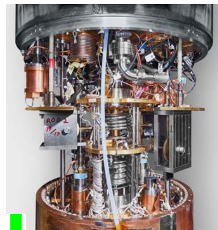
Les scientifiques installent les détecteurs dans le dispositif expérimental d'ADMX (1). La cavité entourée de cuivre est surmontée d'un réservoir d'hélium liquide et de l'électronique de l'expérience (2)
