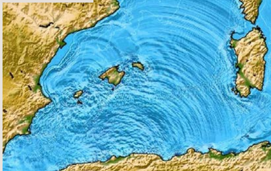
TSUNAMI DÛ AU SÉISME D'ALGER EN 2003
