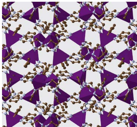
Représentation du ZIF-62 sous sa forme cristalline. Des chercheurs ont développé une méthode pour obtenir en phase amorphe.
