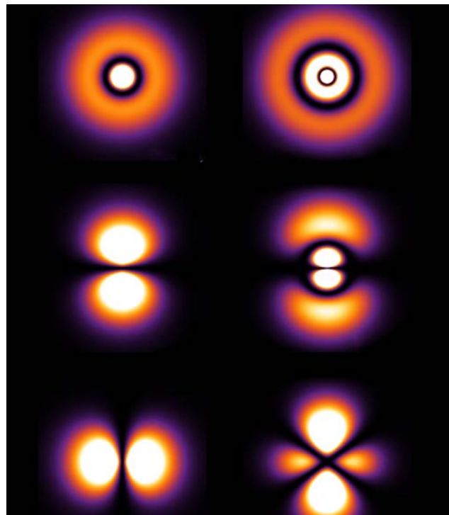
Ces six fonctions d'onde différentes de l'atome d'hydrogène sont représentées ici, dont chacune correspond à une énergie bien définie. La fonction d'onde détermine la probabilité de présence de l'électron (ici, plus la zone est claire, plus il y a de chance que l'électron s'y trouve).
