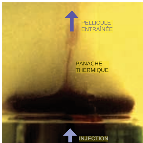
Dans une cuve fermée de un mètre de diamètre, remplie d'eau salée, on injecte un liquide analogue, mais plus dense et plus chaud qui s'élève, entraînant par un panache thermique.
