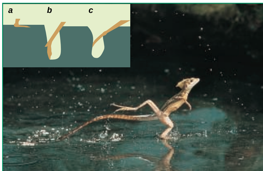
Le basilic, un lézard Sud-américain, court à la surface de l'eau. Ses pas se décomposent en trois phases (en haut). La patte (en marron) frappe d'abord l'eau (a). Puis elle s'enfonce sous l'eau en s'appuyant sur une poche d'air (b). Enfin, la patte est relevée avant que la poche d'air ne disparaisse (c). L'animal est maintenu hors de l'eau principalement grâce aux forces de réaction qui s'exercent lors de la deuxième phase.
