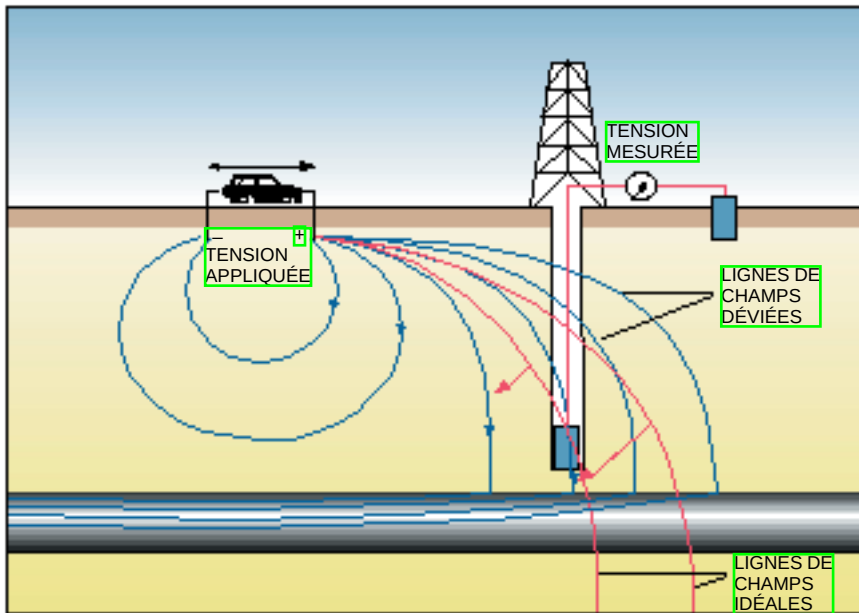
7. LORS DE L'EXPERIENCE de type dipôle-dipôle, une tension électrique était appliquée à la surface du sol à une certaine distance du puits de forage, et le parcours des lignes de champ était mesuré au fond du puits. L'existence de bons conducteurs électriques, dans les couches profondes de la Terre, a été révélée par la déformation des lignes de champ, qui normalement sont circulaires.
