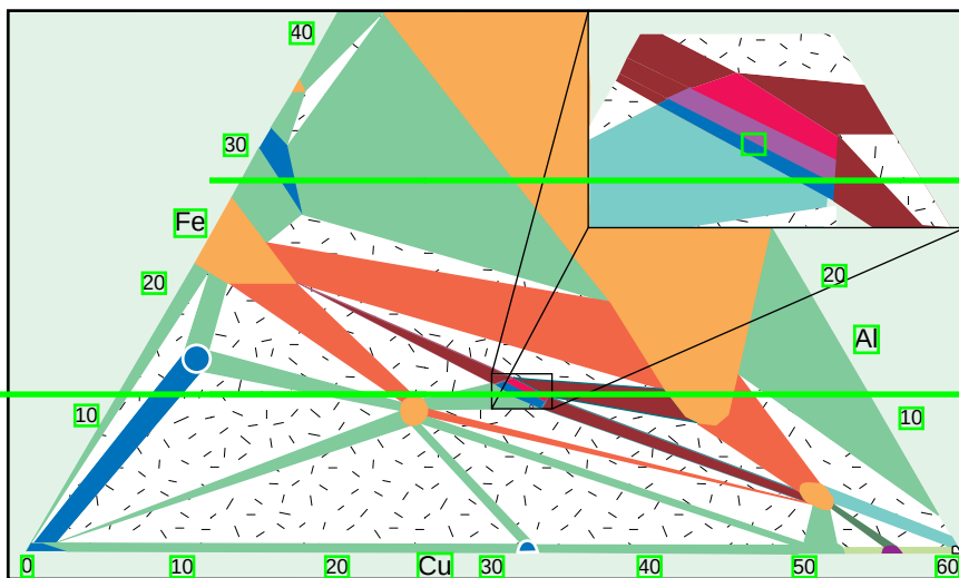
4. COUPE A 700°C du diagramme de phases Al-Cu-Fe montrant en insert un agrandissement de la région de la phase icosaoédrique. Celle-ci se forme dans l'étroite région colorée en rouge qui correspond à une concentration de 1,86 électron par atome. Elle voisine avec des composés cristallins à grande maille (région marquée en bleu) qui possèdent des arrangements atomiques presque identiques. Ce diagramme de phases est la version moderne du diagramme de ce système publié en 1939. Les auteurs soulignaient alors l'existence dans cette région d'une phase nouvelle, impossible à identifier par diffraction des rayons X sur poudre. Les microscopes électroniques n'existaient pas à l'époque...
