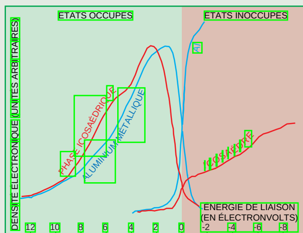
b. Densité des états électroniques de niveau p dans l'aluminium. On a environ quatre fois moins d'électrons au niveau de Fermi dans le composé \text{AlCuFe} icosaoédrique que dans l'aluminium. Dans les états inoccupés, la faible densité des états de conduction de la phase icosaoédrique est visible et la bande de conduction est aplatie.
