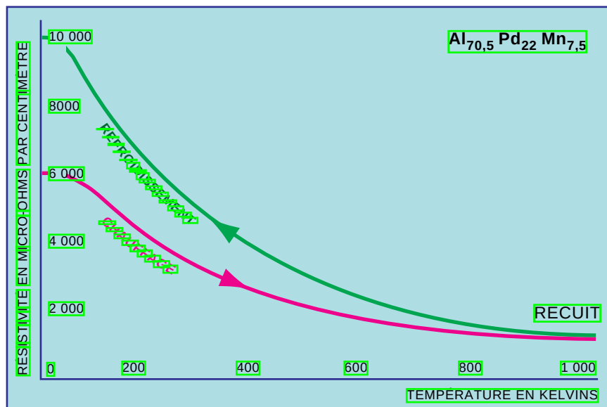
7. LA RESISTIVITE de la phase icosaedrique Al-Pd-Mn est grande à basse température et elle diminue lors du chauffage. Quand on pratique un recuit à haute température pour éliminer les défauts cristallins, la résistivité augmente plus vite lors du refroidissement.
