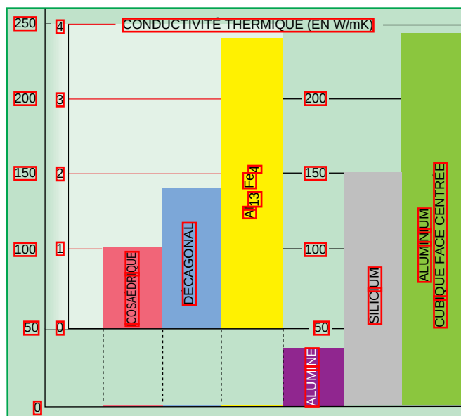
5. CONDUCTIVITES THERMIQUES à la température ambiante comparées entre un métal : l'aluminium, un semiconducteur : le silicium, un oxyde : Al_2O_3 , un composé approximant de la phase décagonale : Al_{13}Fe_4 , une phase décagonale et une phase icosaoédrique polycristallines. La conductivité thermique du quasicristal icosaoédrique est 250 fois plus faible que celle de l'aluminium.
