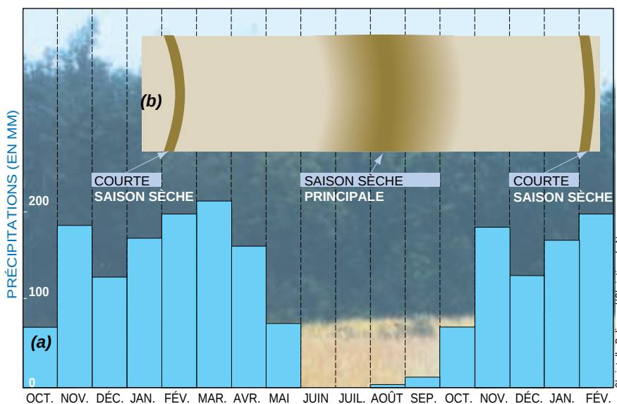
L'alternance de saisons sèches et de saisons des pluies, visible sur l'histogramme des précipitations (en bleu (a)), est responsable de la formation de cernes dans un tronc d'okoumé (b).
