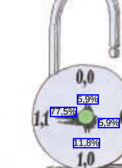
L'ALGORITHME DE GROVER DISTINGUE LE BON ÉTAT
