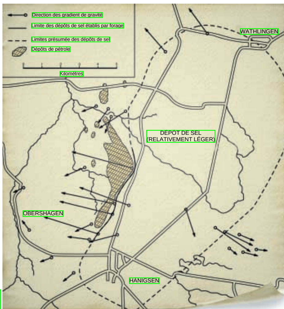
2. UNE ETUDE GEOPHYSIQUE réalisée en 1917 près de Hanovre, à l'aide d'une balance de torsion, prouva que l'on pouvait repérer des dépôts de sel souterrains grâce à la gradiométrie gravitationnelle. Ces formations salifères, moins denses que les roches environnantes, indiquent généralement que des gisements de gaz et de pétrole (zones hachurées) sont situés à proximité.
