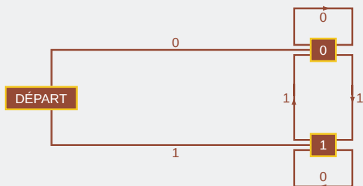
AUTOMATE POUR LA SUITE DE THUE-MORSE = 0,1101001100101101001101001\dots
