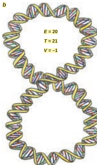
2. Cette boucle d'ADN a des caractéristiques de vrillage, de tortillement et d'enroulement qui vérifient l'équation E = V + T , que la molécule soit dans un état relâché (a) ou surenroulé (b et c).
