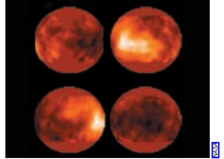
Vues de la surface de Titan photographié en infrarouge par Hubble. Les zones les plus brillantes, seraient des régions de relief élevé.
