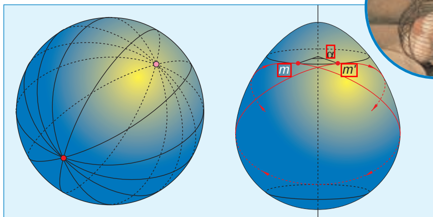
7. SUR UNE SPHERE (à gauche), toutes les trajectoires d'une particule lancée sur la surface sans frottements et sans gravité sont des géodésiques périodiques : ce sont les grands cercles. Sur une surface de révolution (à droite), telle celle d'un œuf, les trajectoires (en rouge) sont des géodésiques périodiques pourvu qu'à partir d'un point m d'un parallèle quelconque (en noir), elles repassent sur ce même parallèle par un point m' décalé de m d'un angle \alpha en rapport rationnel avec 2\pi .
