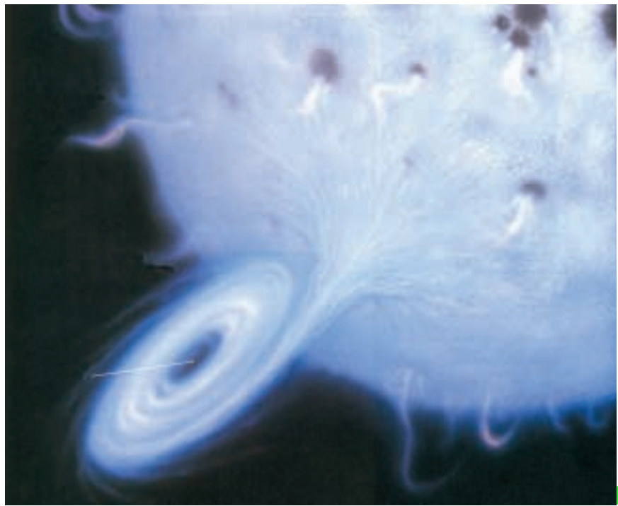
6. A LA FIN DE LEUR EXISTENCE, certaines étoiles peuvent donner naissance à des trous noirs. Si ces objets compacts font partie d'un système double, leur attraction gravitationnelle immense leur permet d'arracher du gaz à la surface de leur compagnon. Le gaz s'accumule en tournoyant dans un disque d'accrétion avant de disparaître finalement dans le trou noir.
