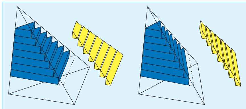
5. EN DÉCOUPANT DEUX TÉTRAÈDRES de même hauteur et de même aire de base en tranches, on montre qu'ils ont le même volume. Les tranches sont composées d'un prisme (en bleu) et d'un bout restant (en jaune). Dans chaque tétraèdre, les prismes du même niveau, ont un volume égal. Lorsque le nombre de prismes est infini, le volume des bouts restants est égal à zéro : les tétraèdres ont donc même volume.
