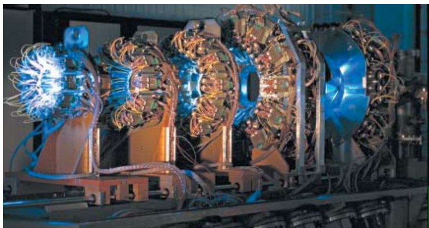
8. LE SYSTÈME INDRA détecte les protons et toutes les particules chargées.
