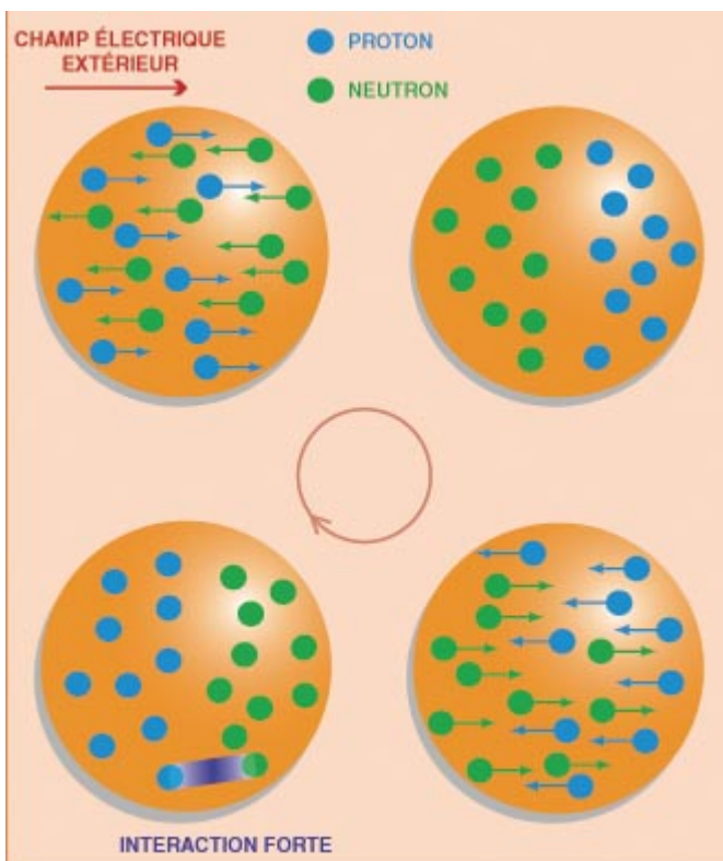
1. LA RÉSONANCE DIPOLAIRE fut la première résonance géante découverte. Les protons (en bleu) oscillent en opposition de phase avec les neutrons (en vert).
