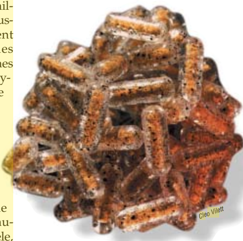
5. CE MODÈLE DE POUSSIÈRE DE COMÈTE, élaboré par l'auteur, montre 100 gros grains qui forment un amas peu dense de trois micromètres de diamètre. Riche en composés organiques, ces agrégats ont peut-être été des germes de vie sur Terre.
