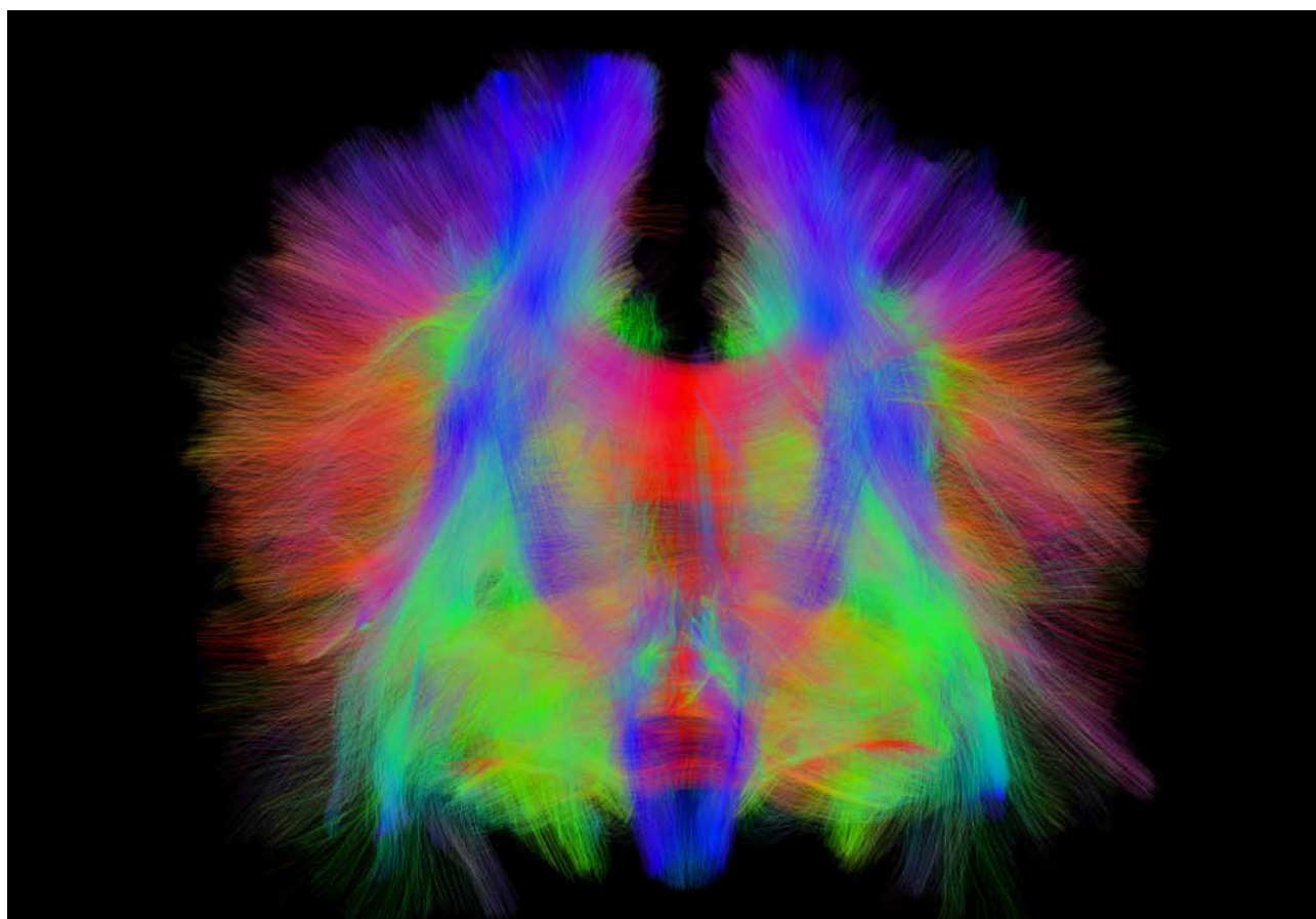
1. LA CONNECTOMIQUE a pour objectif d'établir la carte de toutes les connexions neuronales du cerveau. L'image ci-dessus représente ainsi les voies suivies par les fibres de la substance blanche, composée essentiellement d'axones. Dans cette reconstruction obtenue par la technique d'IRM de diffusion, les couleurs codent l'orientation des fibres : rouge pour la direction gauche-droite, vert pour la direction avant-arrière et bleu pour la direction dessus-dessous.
