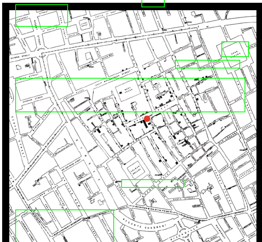
LA CARTOGRAPHIE DES CAS DE CHOLÉRA (en noir) en 1854 à Londres a amené le médecin John Snow jusqu'à la source de la maladie : une pompe publique, dont l'eau avait été contaminée par des matières fécales (point rouge). Cette méthode est toujours utilisée aujourd'hui, mais le réseau de détecteurs de pathogènes proposé par l'auteur permettrait de déterminer l'origine d'une épidémie bien plus vite.
