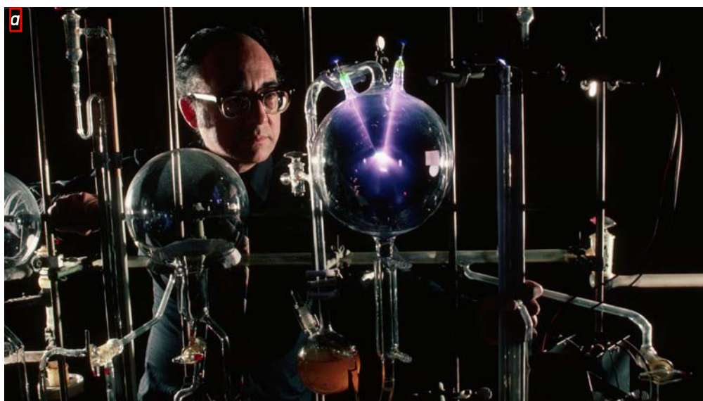
Pour identifier les réactions chimiques dans l'expérience de Stanley Miller [a], A. Marco Saitta et Franz Saija ont modélisé le processus. Ils montrent que les molécules d'eau, d'ammoniac et de monoxyde de carbone [b] interagissent et forment du formamide [c] puis de la glycine [d], l'acide aminé le plus simple.
