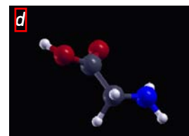
Pour identifier les réactions chimiques dans l'expérience de Stanley Miller [a], A. Marco Saitta et Franz Saija ont modélisé le processus. Ils montrent que les molécules d'eau, d'ammoniac et de monoxyde de carbone [b] interagissent et forment du formamide [c] puis de la glycine [d], l'acide aminé le plus simple.
