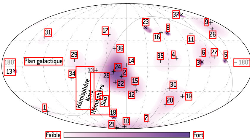
Probabilité d'une source ponctuelle à l'origine du signal LA CARTE DES NEUTRINOS de haute énergie établie par IceCube répertorie la provenance des particules (qui sont numérotées). On note une accumulation de neutrinos proche du centre galactique. L'intensité de la couleur violette reflète la probabilité qu'une source ponctuelle soit à l'origine du signal. Certains neutrinos, très éloignés du plan galactique, sont originaires d'au-delà de la Voie lactée.
