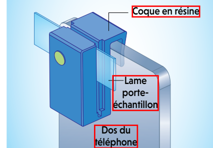
DISPOSITIF VU DU DESSUS
