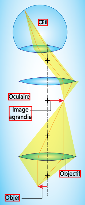
PRINCIPE D'UN MICROSCOPE
