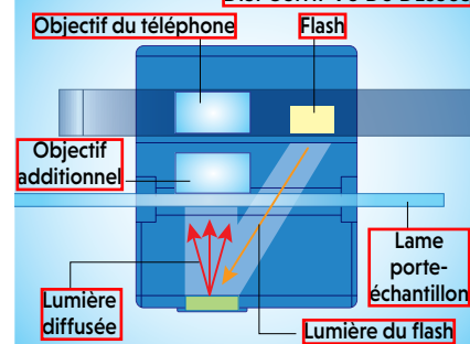
DISPOSITIF VU DU DESSUS
