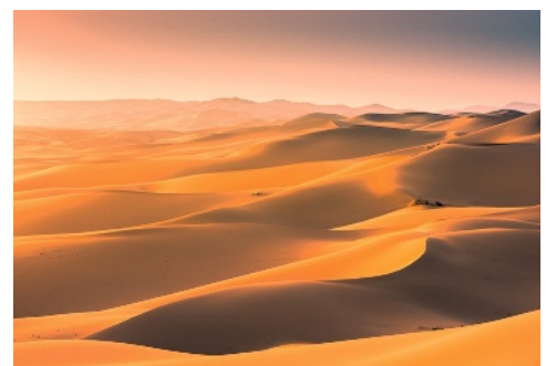
Isolée, une dune plus petite avance plus vite, mais des dunes proches subissent un couplage qui les écarte.
