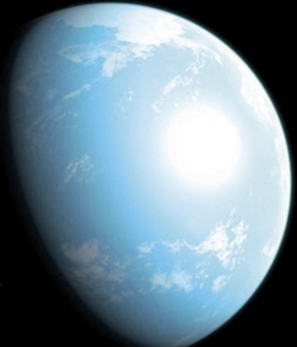
Vue d'artiste de l'exoplanète GJ 357 d, distante de 31 années-lumière.
